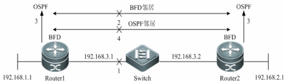
图 3-3 BFD 检测
