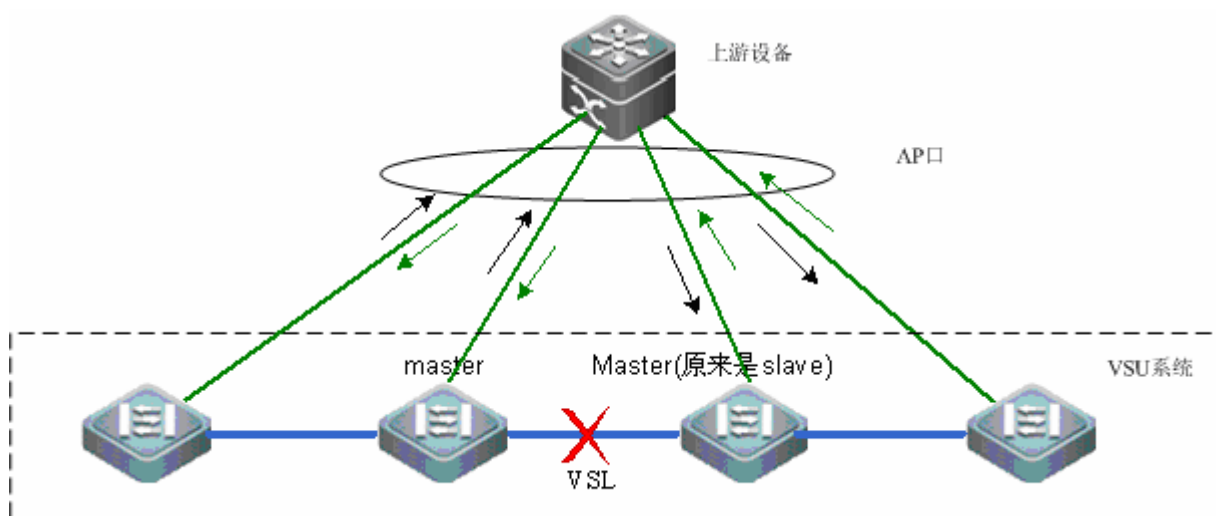
图 5-12 基于聚合口双主机检测
