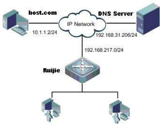
图 3-2 动态域名解析配置组网图
