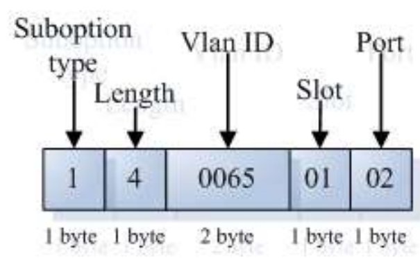
图 2-4 Agent Remote ID
