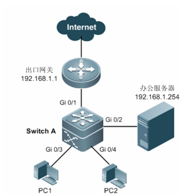
图 10-1 防网关 ARP 欺骗典型拓扑
