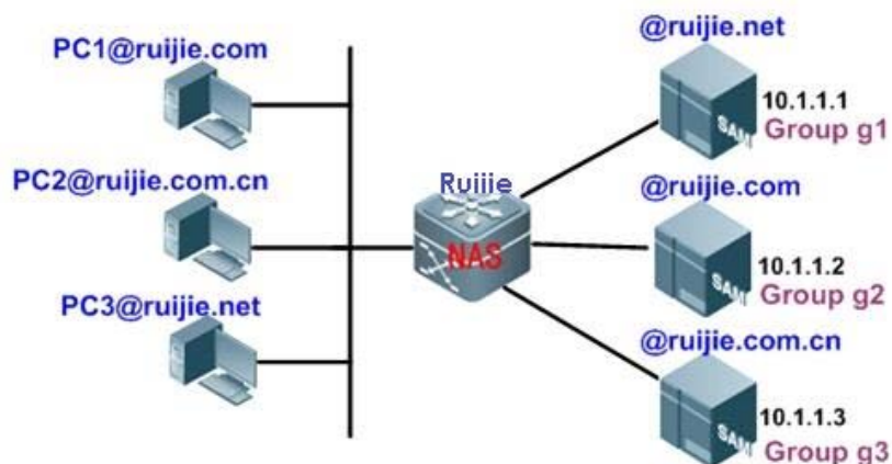
图 1-4 AAA 多域认证应用图
