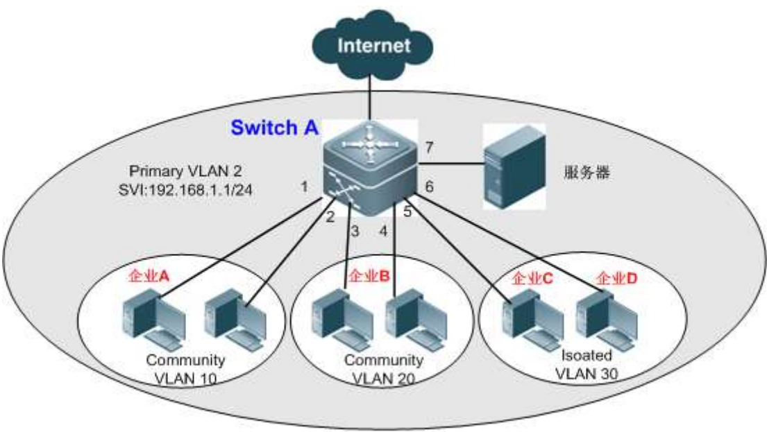
图 6-2 PVLAN 单台设备三层应用拓扑
