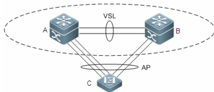
图 5-13 跨设备聚合端口
