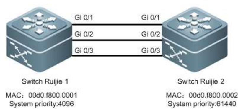
图 4-2 LACP 链路聚合
