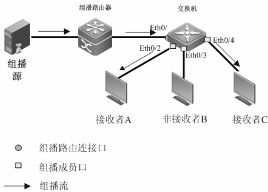
图 1-2 IGMP Snooping 的两类端口
