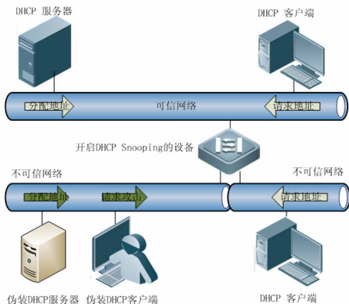
图 9-4 通过 DHCP Snooping 进行保护的网路
