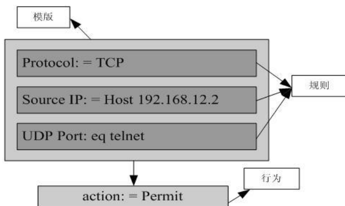
图 1-2 对 ACE: permit tcp host 192.168.12.2 any eq telnet 的分析
