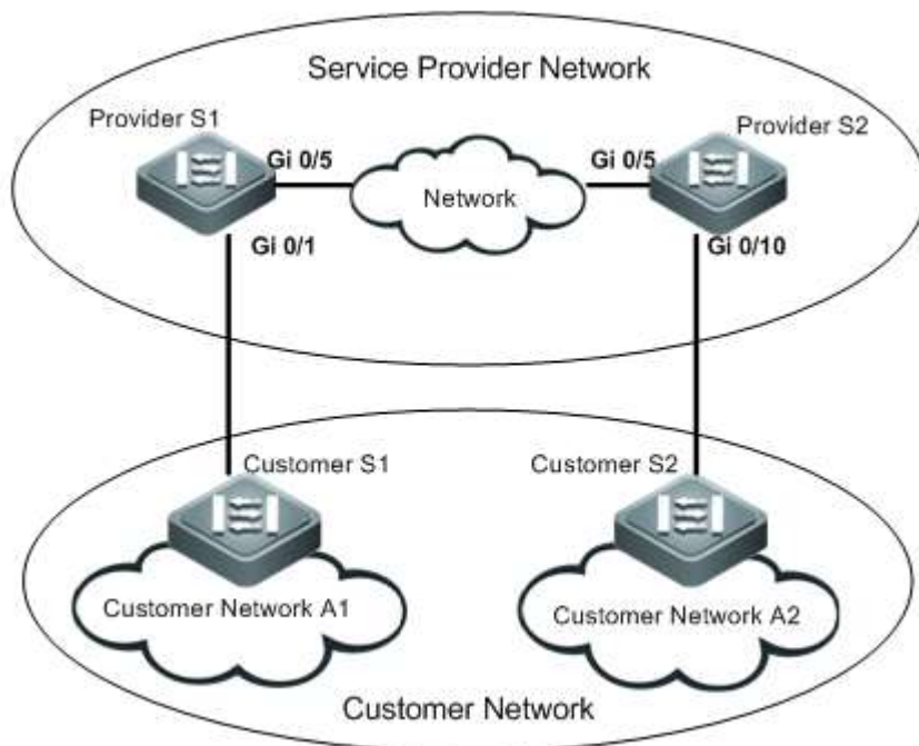
图 11-5 BPDU Tunnel 应用拓扑图
