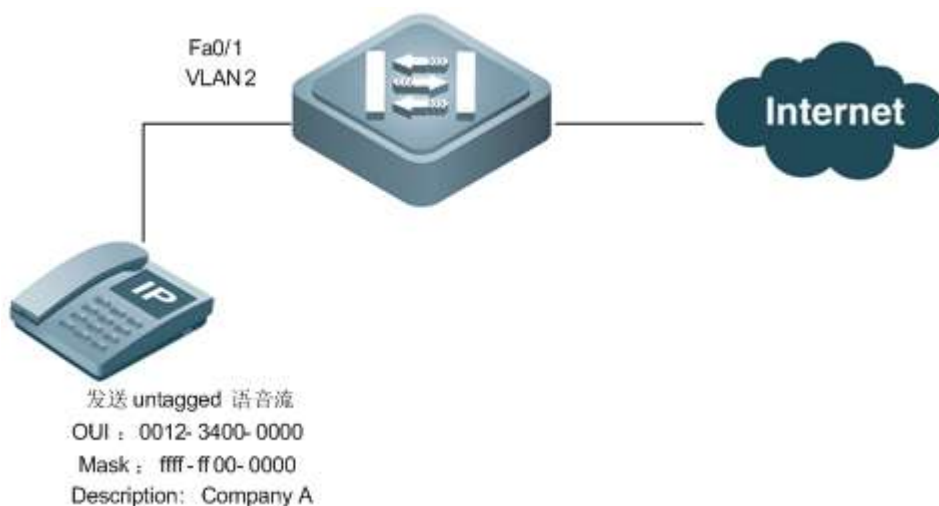
图 7-3 Voice VLAN 手动模式配置组网图
