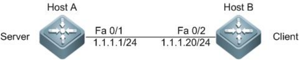
图 3-1 NTP 客户端/服务器模型
