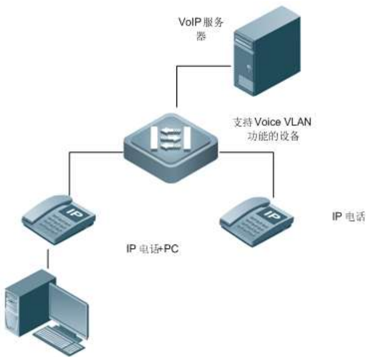
图 7-1 Voice VLAN 基本组网图
