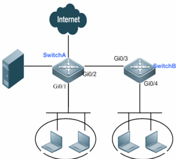
图 1-5 RLDP 应用拓扑图
