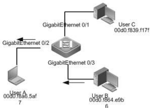
图 2-5 以太网交换机 MAC 地址表二
