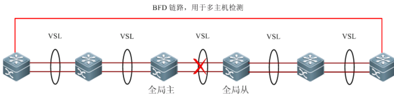
图 5-11 基于 BFD 的多主机检测
