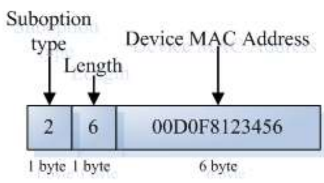
图 2-4 Agent Remote ID
