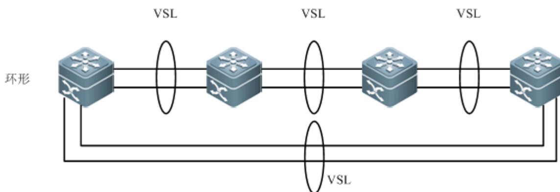
图 5-7 环形拓扑
