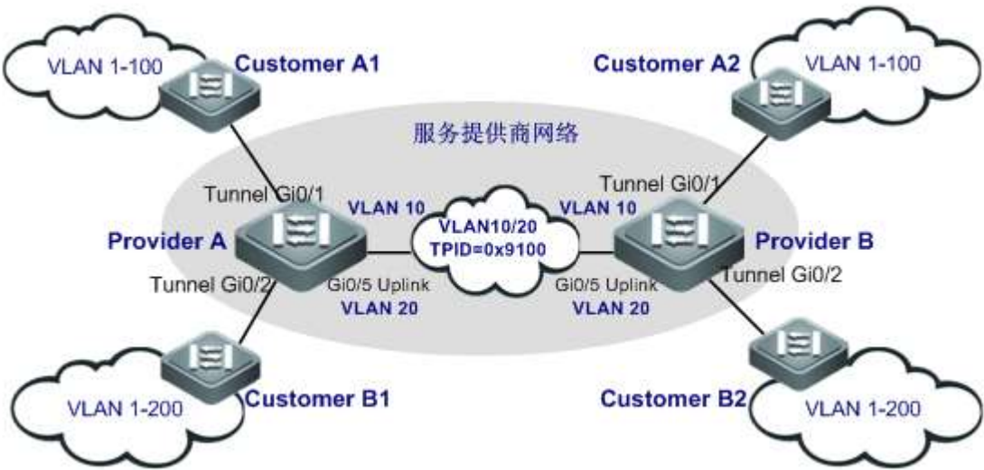
图 11-4 基本 QinQ 实现二层 VPN 业务应用拓扑
