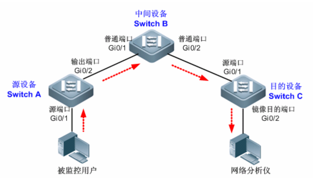
图 6-2 RSPAN 的应用拓扑
