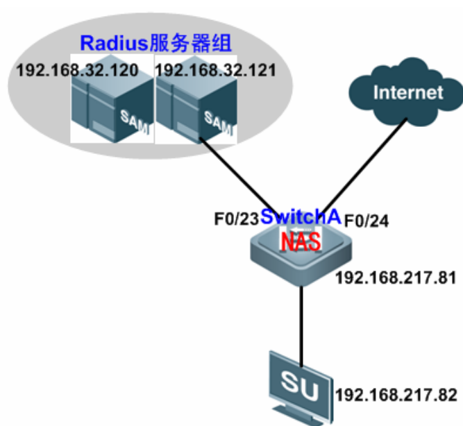
图 2-14 基于端口的用户 1X 认证及 IP 授权应用拓扑图
