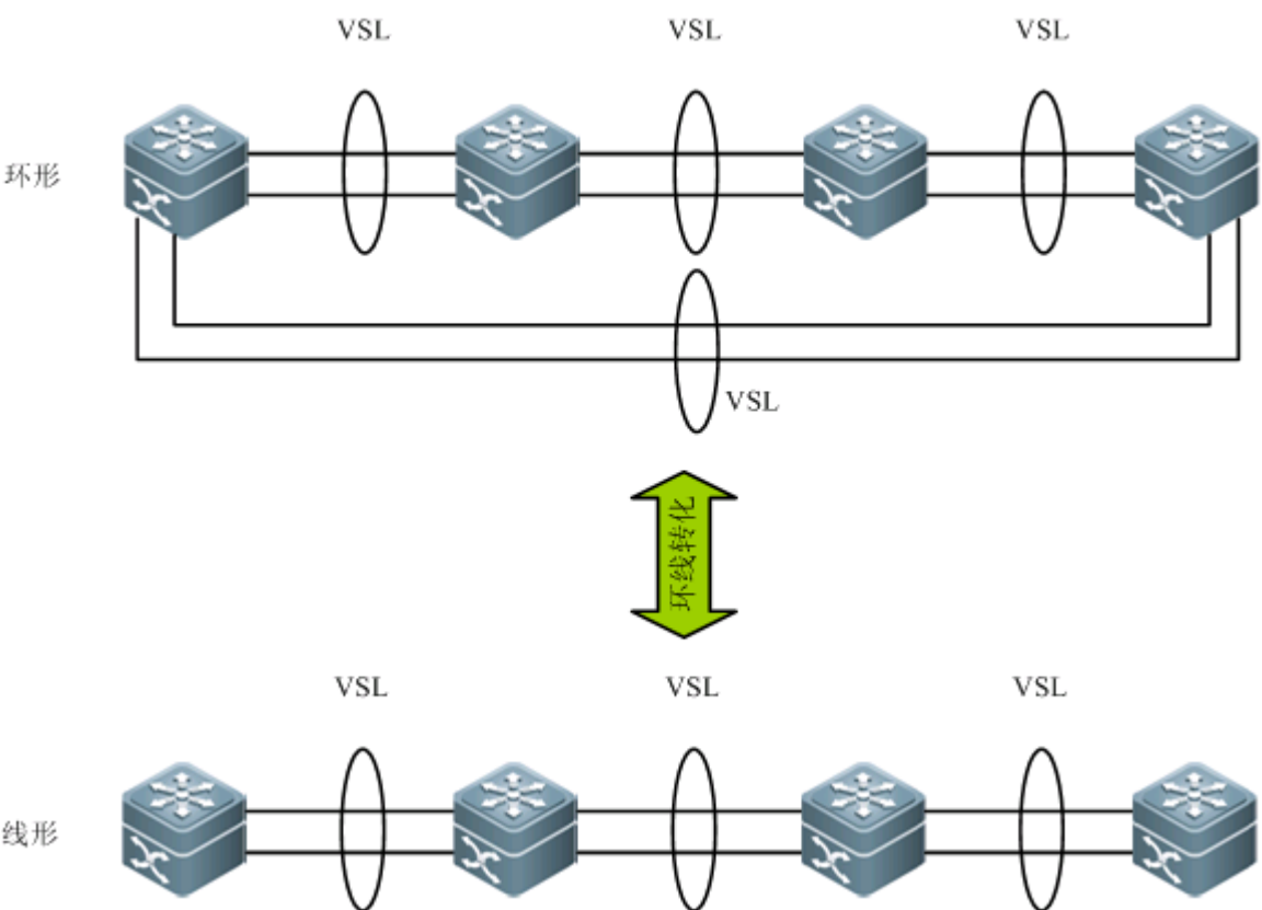
图 5-8 环转线、线转环
