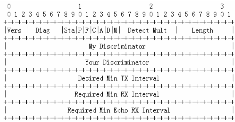
图 3-1 BFD 控制报文（版本 1）格式
