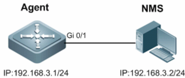
图 1-6 SNMPv3 应用拓扑
