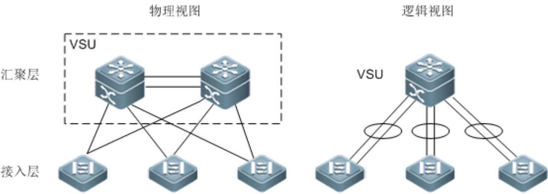
图 5-3 汇聚层的 VSU
