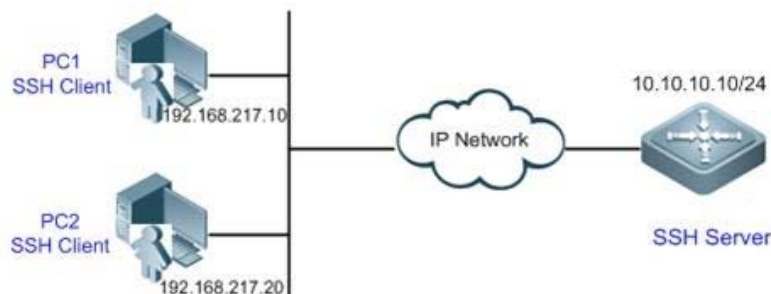
图 3-9 SSH 本地线路口令保护组网图
