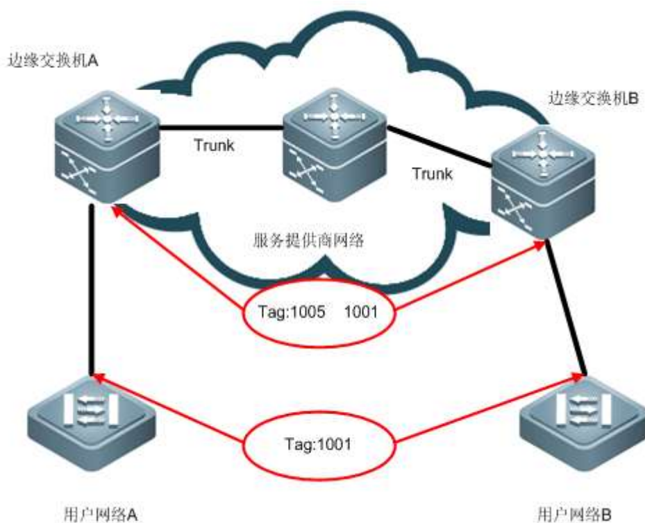
图 11-1 QinQ 示意图
