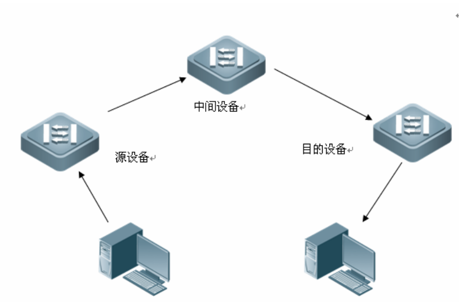
图 6-1 RSPAN 典型应用拓扑图
