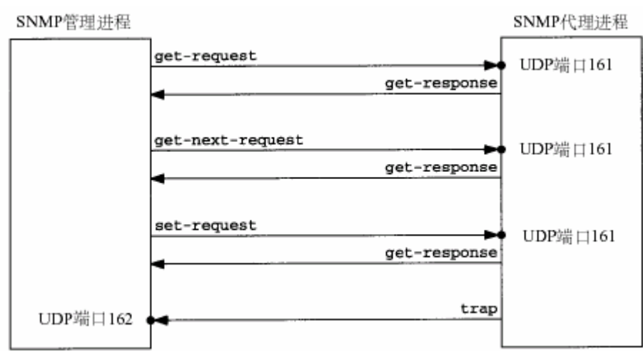
图 1-3 SNMP 的报文类型
