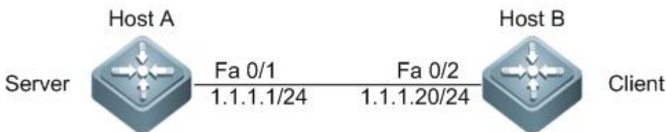
图 3-2 NTP 客户端/服务器模型
