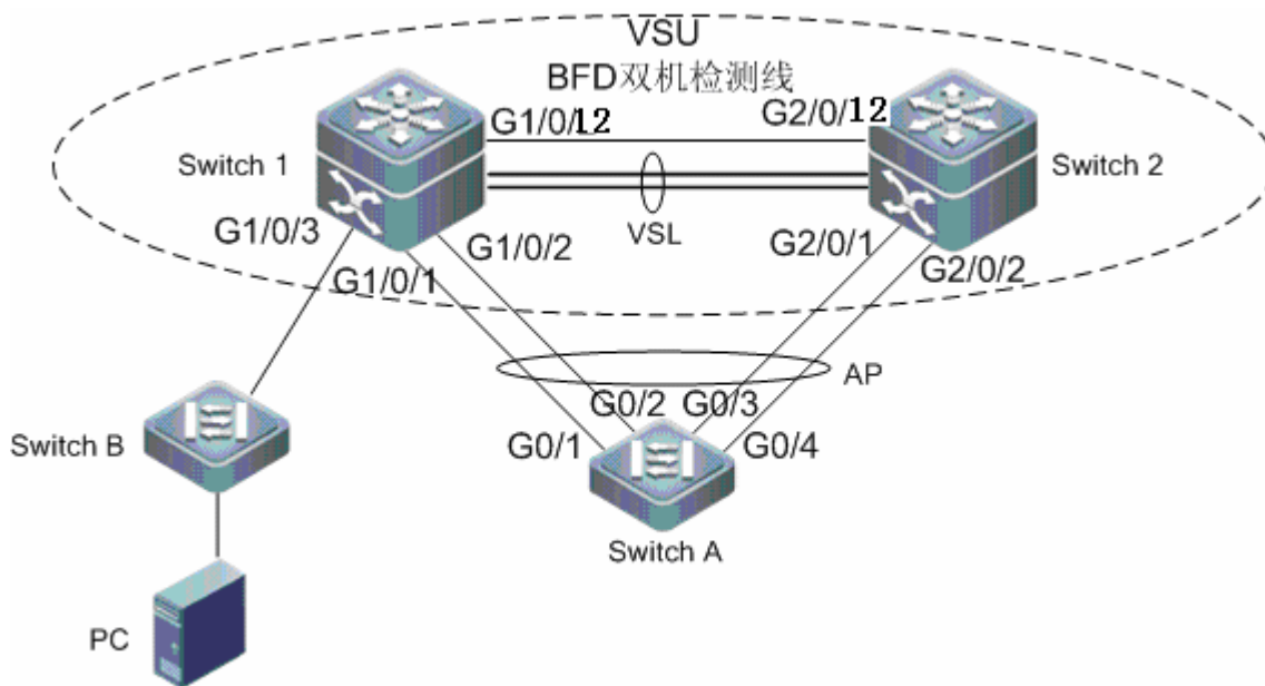
图 5-15 VSU 组网拓扑
