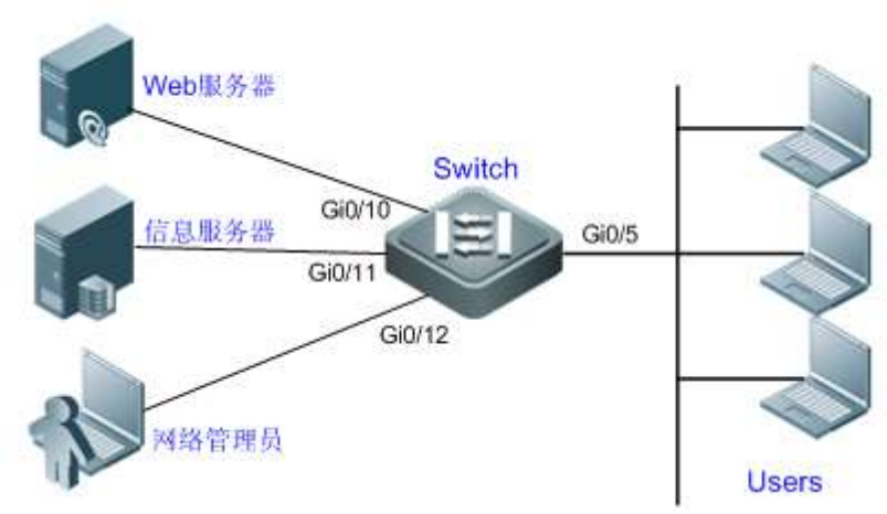
图 2-7 静态 MAC 地址应用组网拓扑
