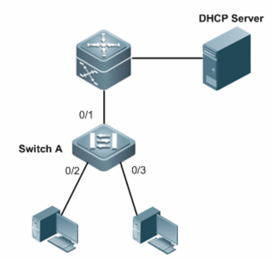
图 9-5 DHCP 部署环境
