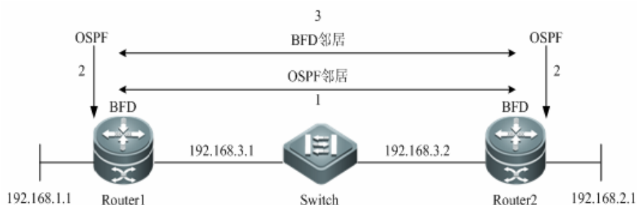
图 3-2 建立 BFD 会话
