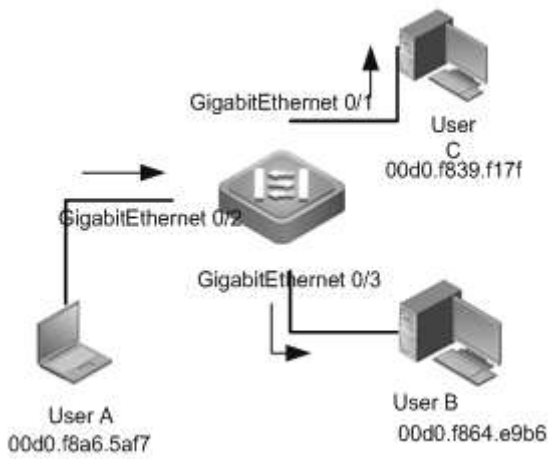
图 2-3 以太网交换 MAC 地址表一
