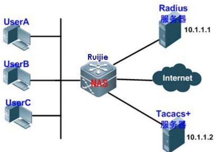
图 1-3 AAA 典型应用图
