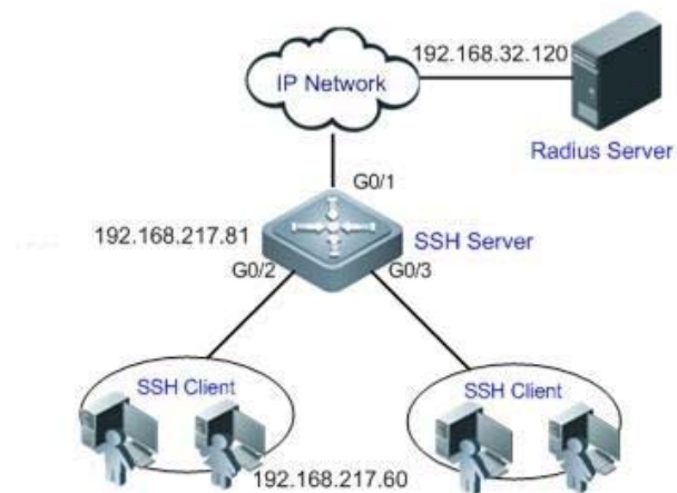
图 3-13 SSH AAA 认证组网图
