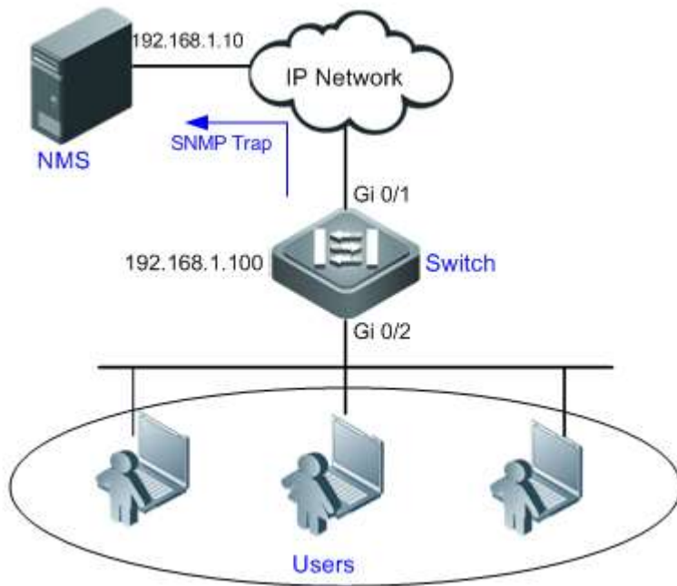
图 2-8 MAC 地址变化通知组网拓扑图
